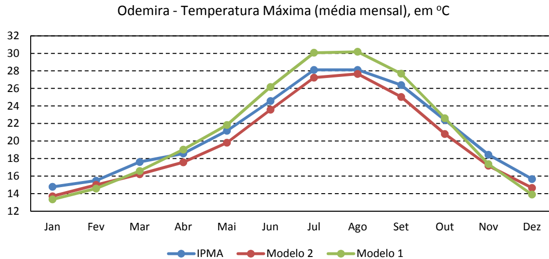
Figura 6 - Comparação entre os valores observados (IPMA) e os modelados para o clima presente (1976-2005)
