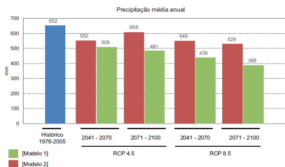
Figura V.1 – Precipitação média anual observada no período entre 1976-2005, e projeções até ao final do século. Os dados são relativos a dois modelos climáticos e dois cenários (RCP4.5 e RCP8.5).
