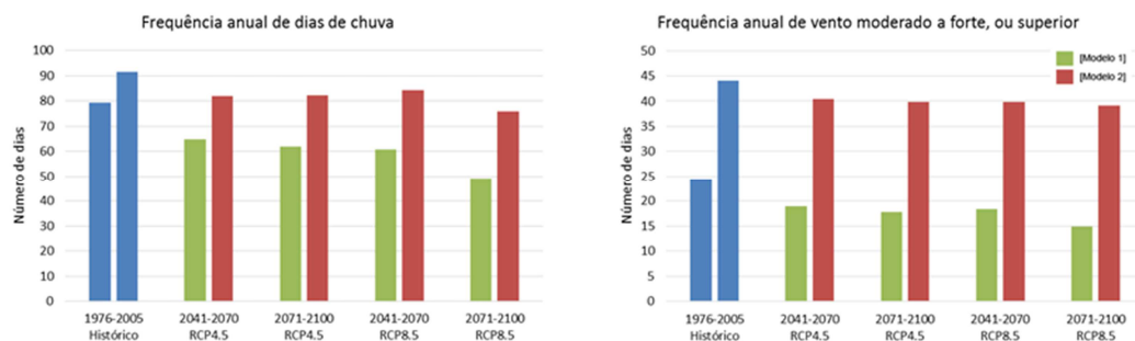
Figura V.2 – Projeções das variáveis climáticas para dois modelos e dois cenários (RCP4.5 e RCP8.5), até ao final do século, relativas ao município de Odemira. A barra azul à esquerda refere-se ao histórico do modelo 1, e a barra azul à direita refere-se ao histórico do modelo 2.
