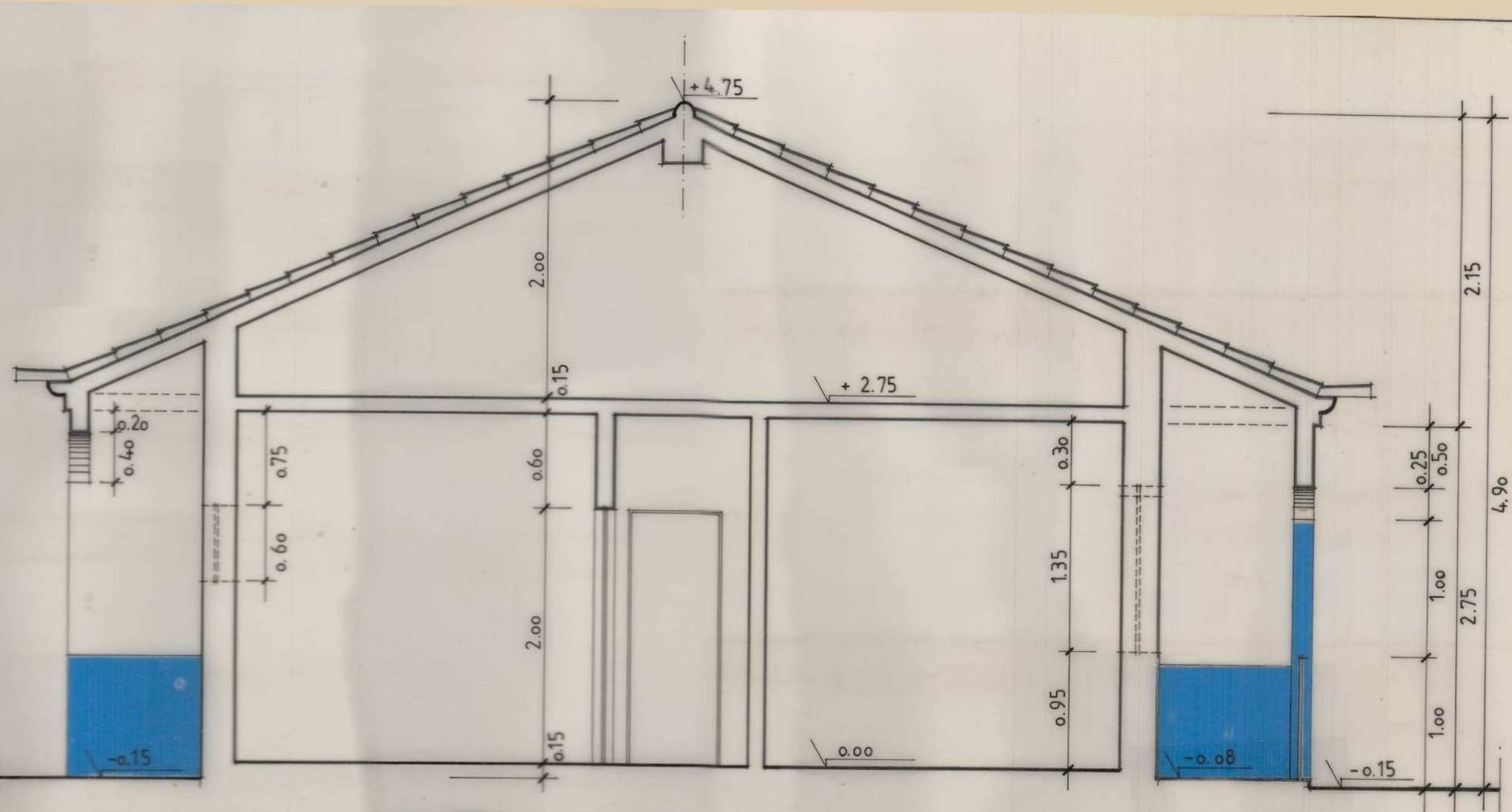
Corte AB
