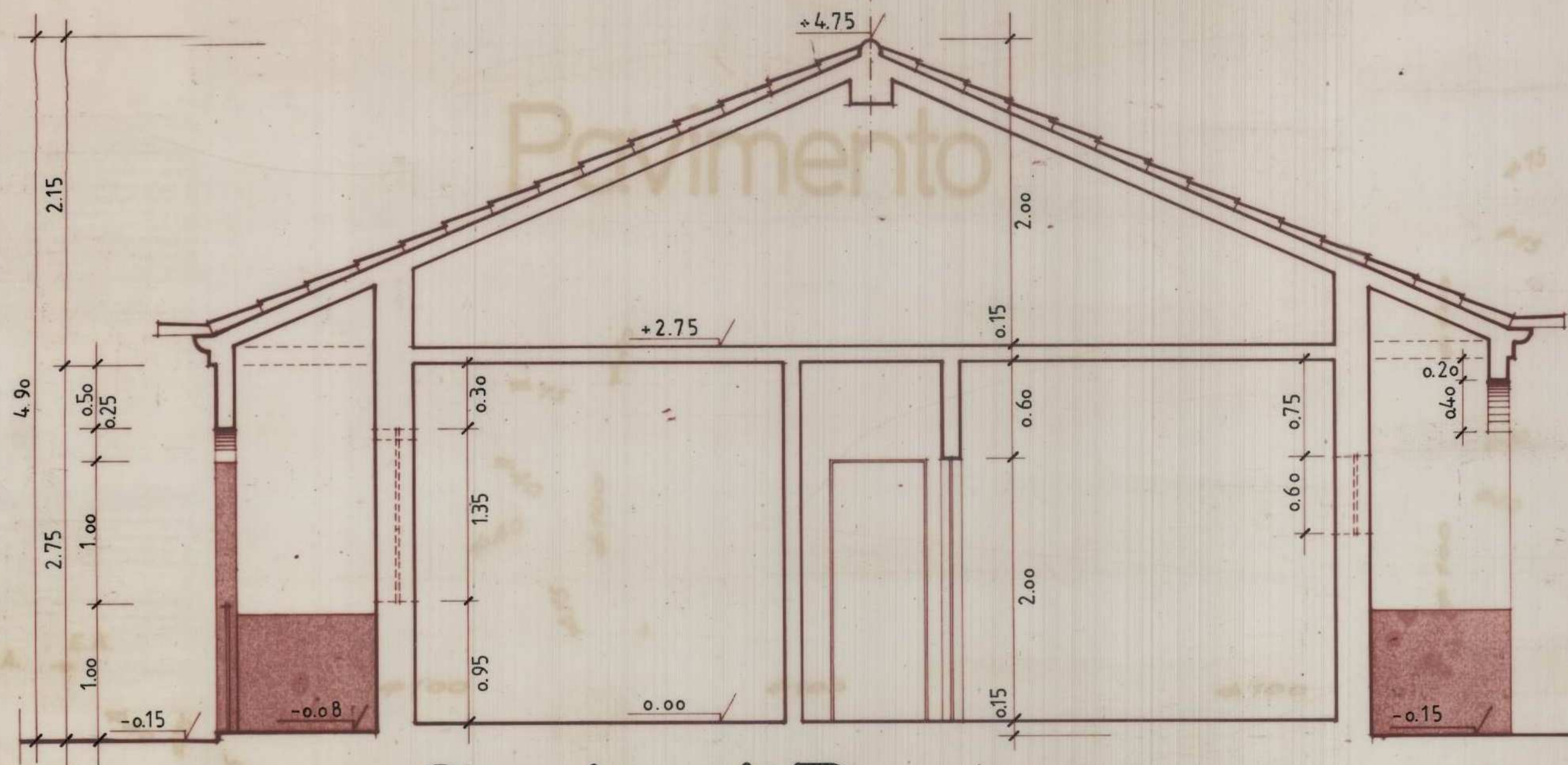
Corte AB
