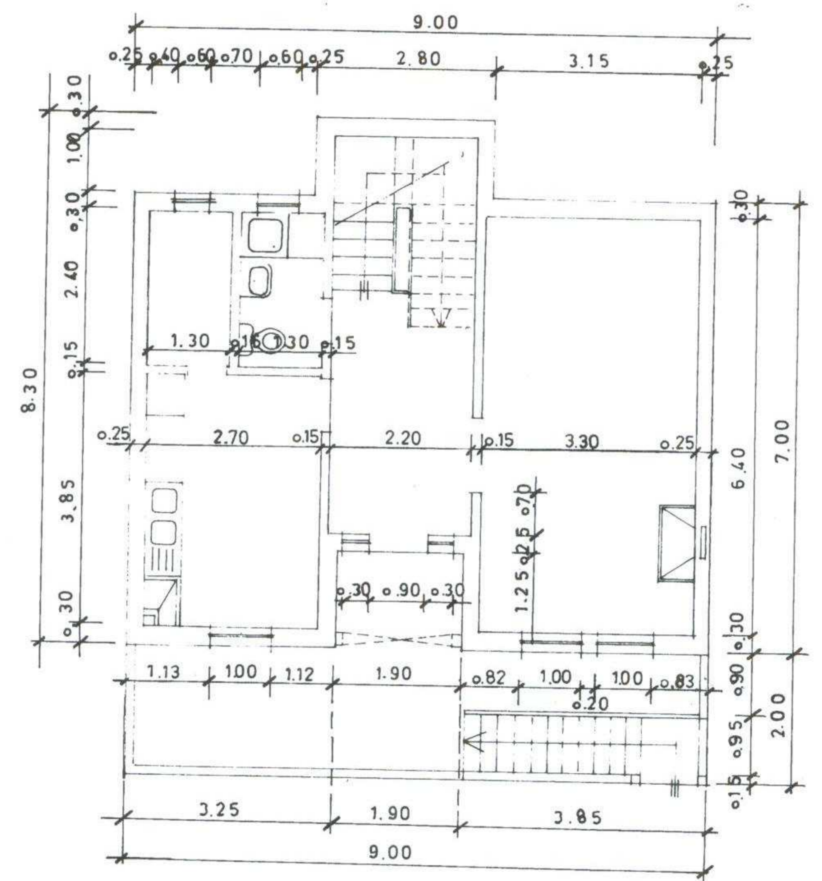
PISO 1
