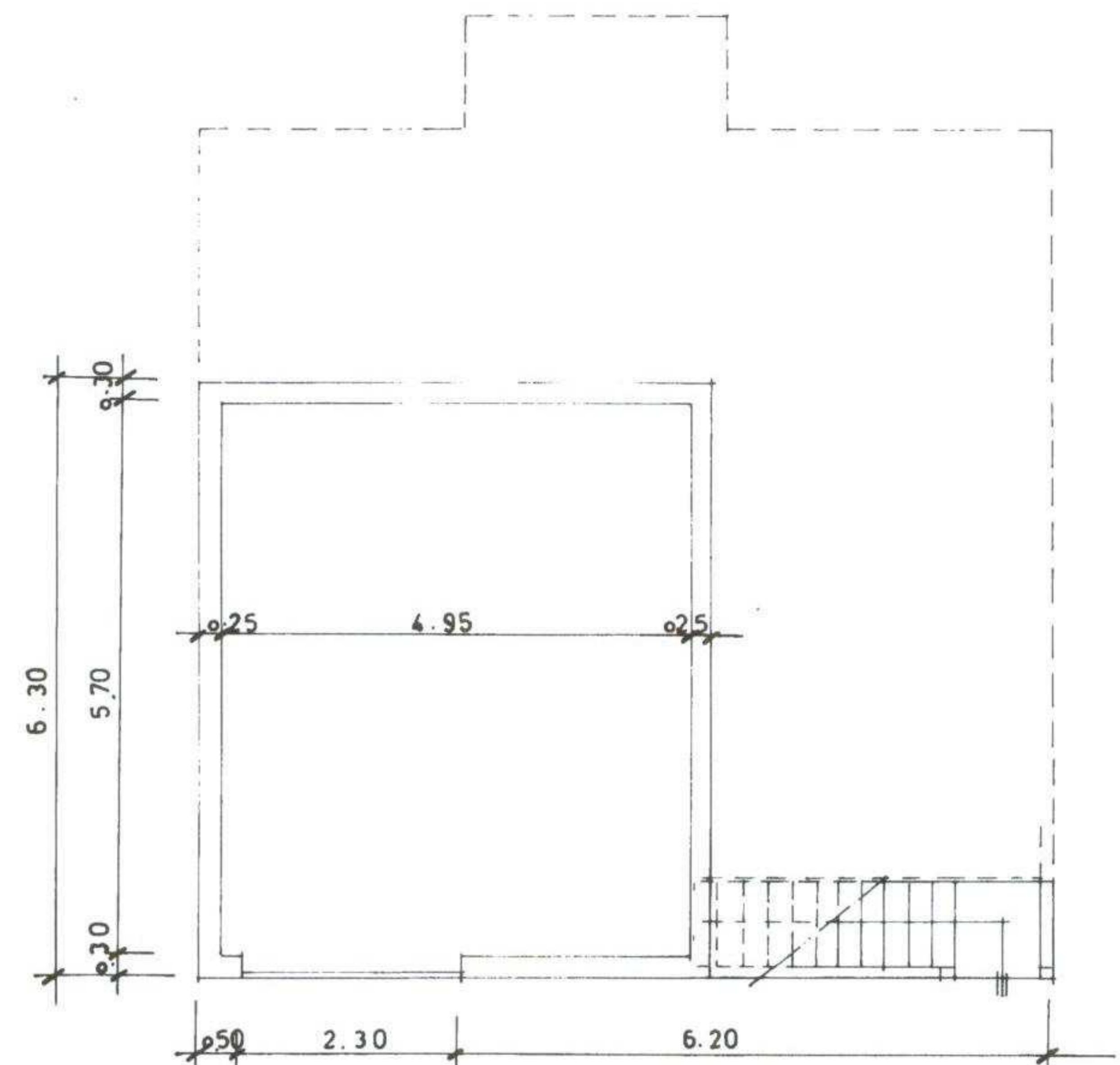
PISO 0
