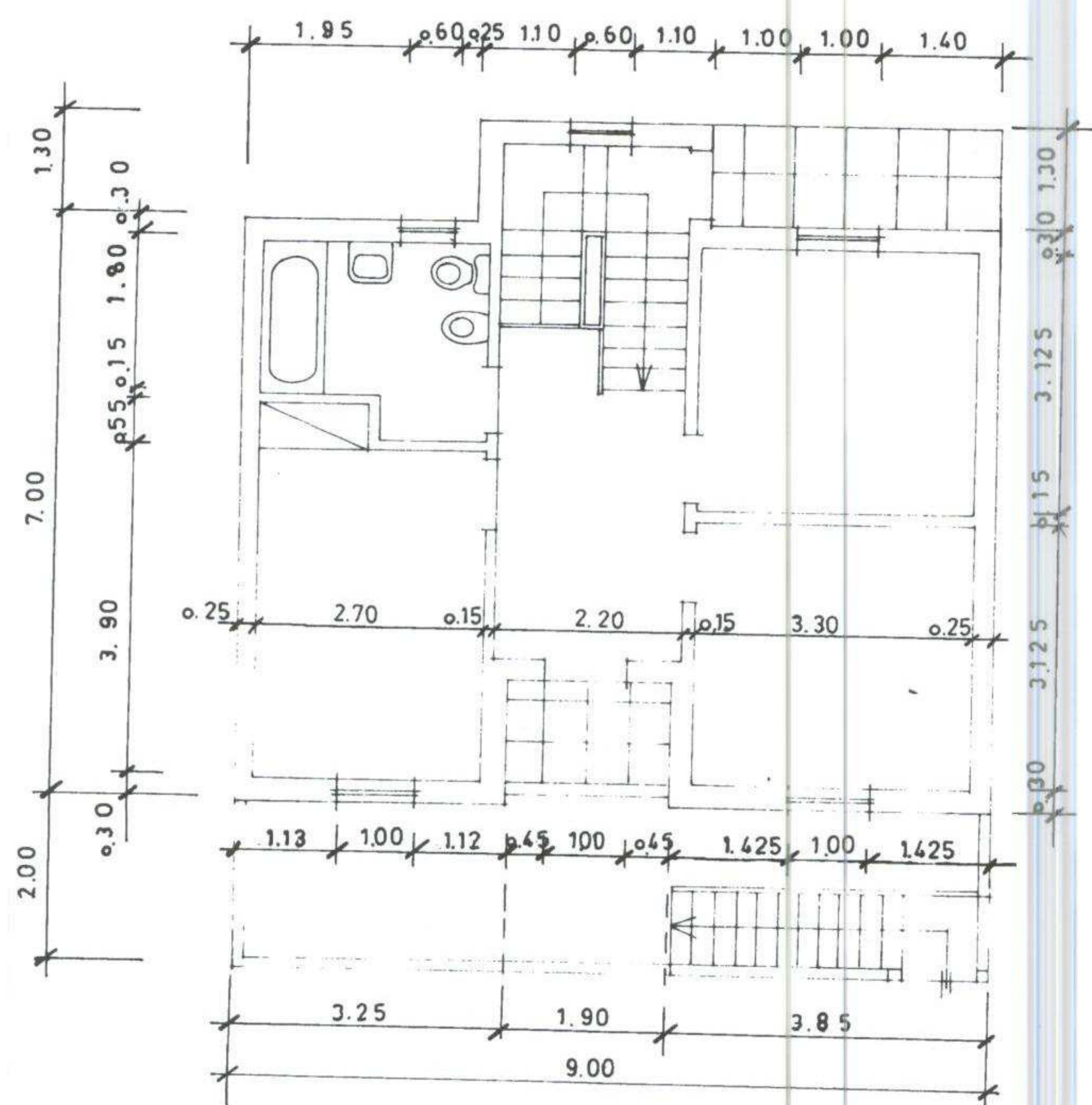
PISO 2
