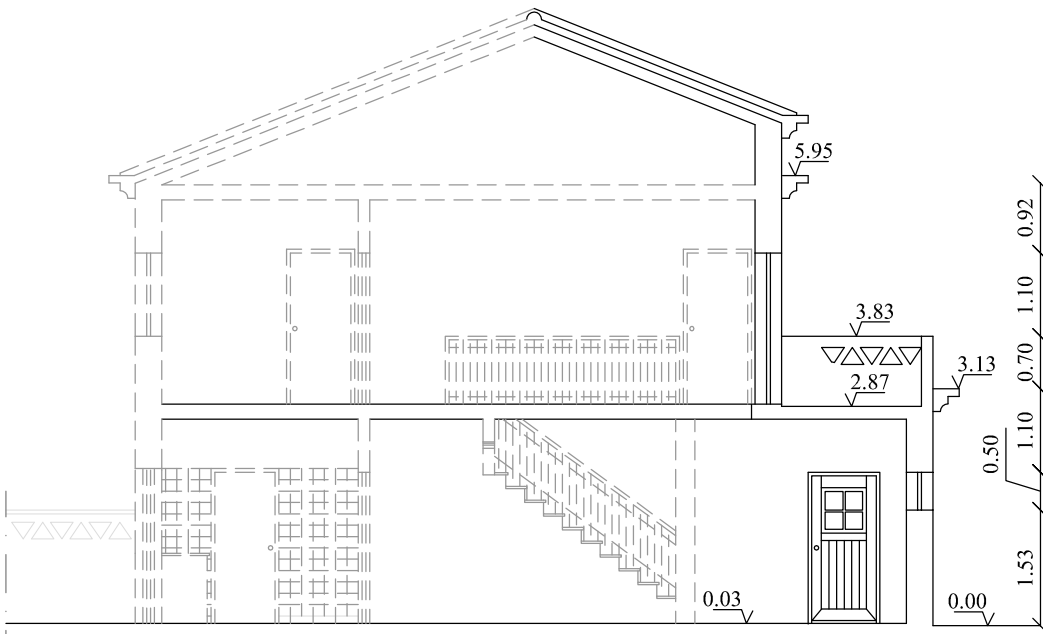
CORTE XX' VERSÃO DIREITA
