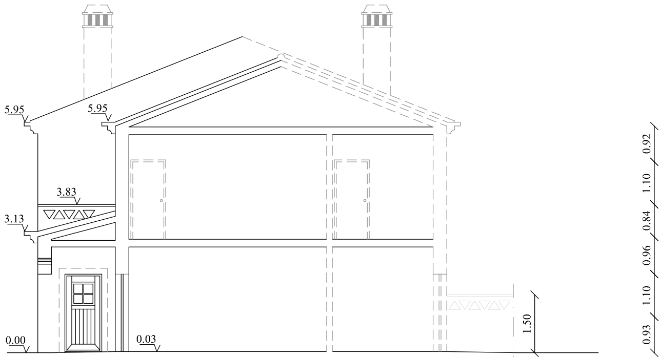
CORTE YY' VERSÃO DIREITA
