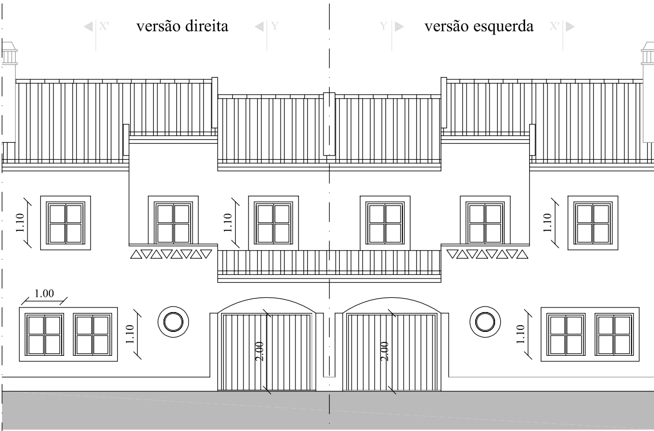
ALÇADO PRINCIPAL DE CONJUNTO
