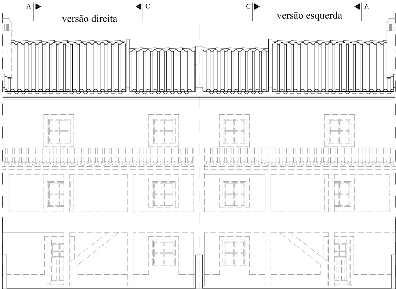
ALÇADO POSTERIOR DE CONJUNTO
