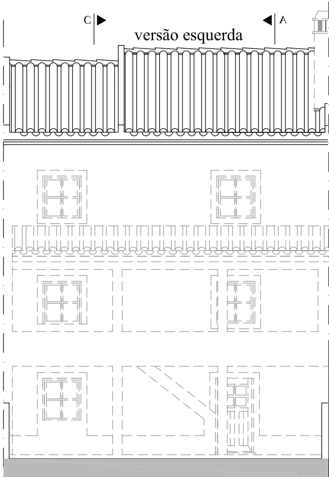
ALÇADO POSTERIOR VERSÃO ESQUERDA
