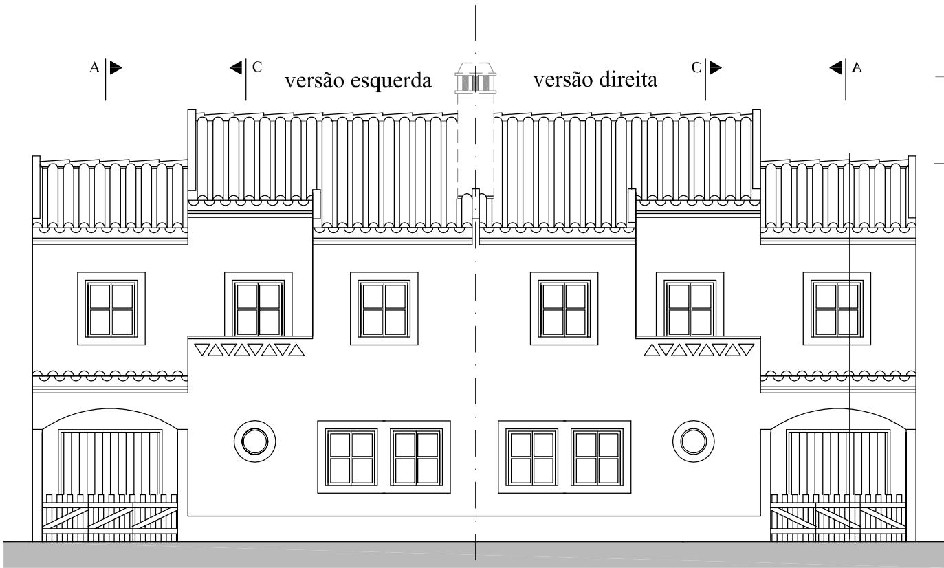
ALÇADO PRINCIPAL DE CONJUNTO
