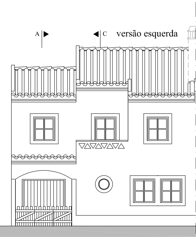
ALÇADO PRINCIPAL VERSÃO ESQUERDA
