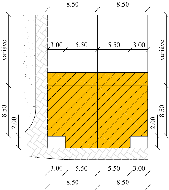
IMPLANTAÇÃO DA CONSTRUÇÃO
